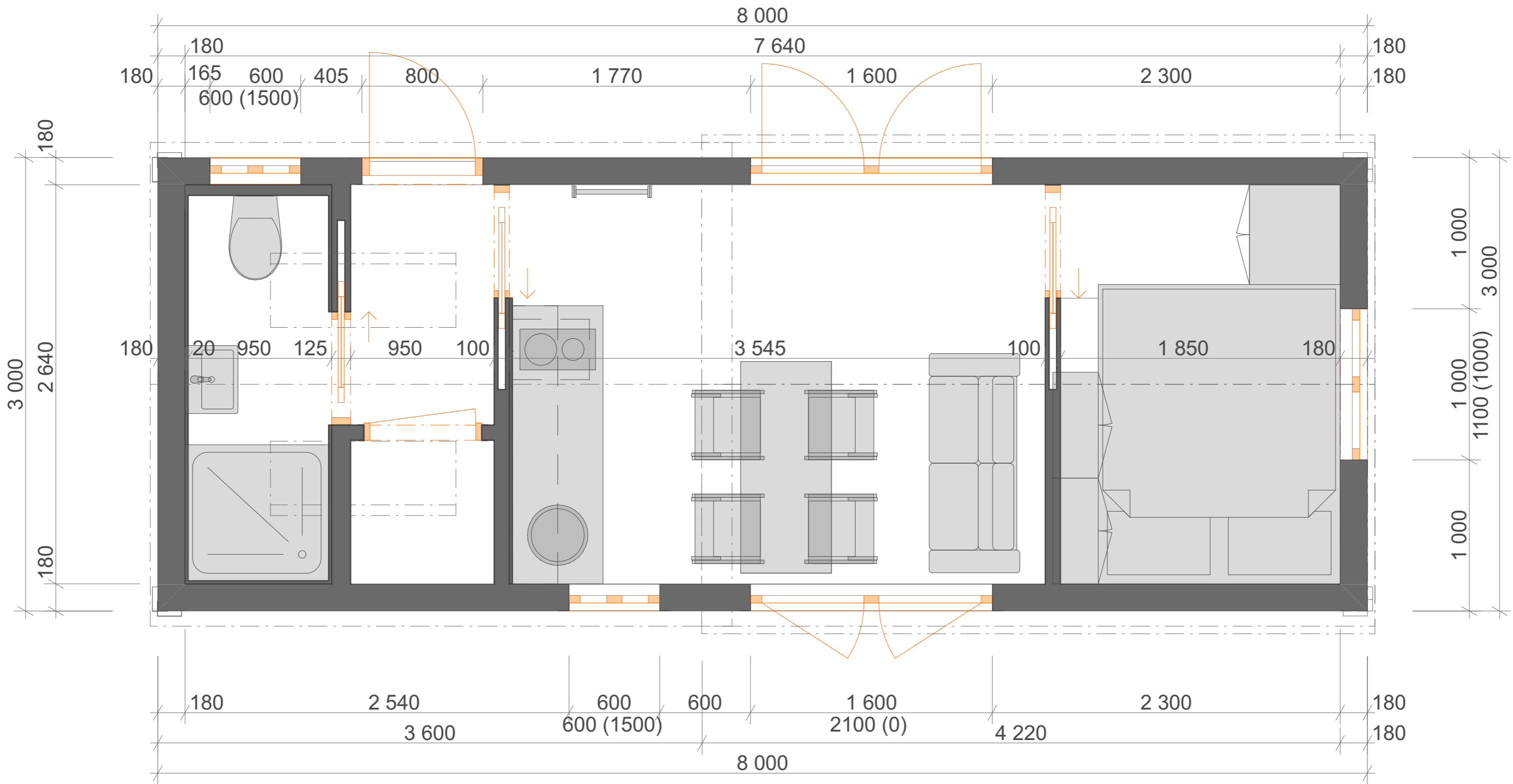
Schéma půdorysného rozvržení
