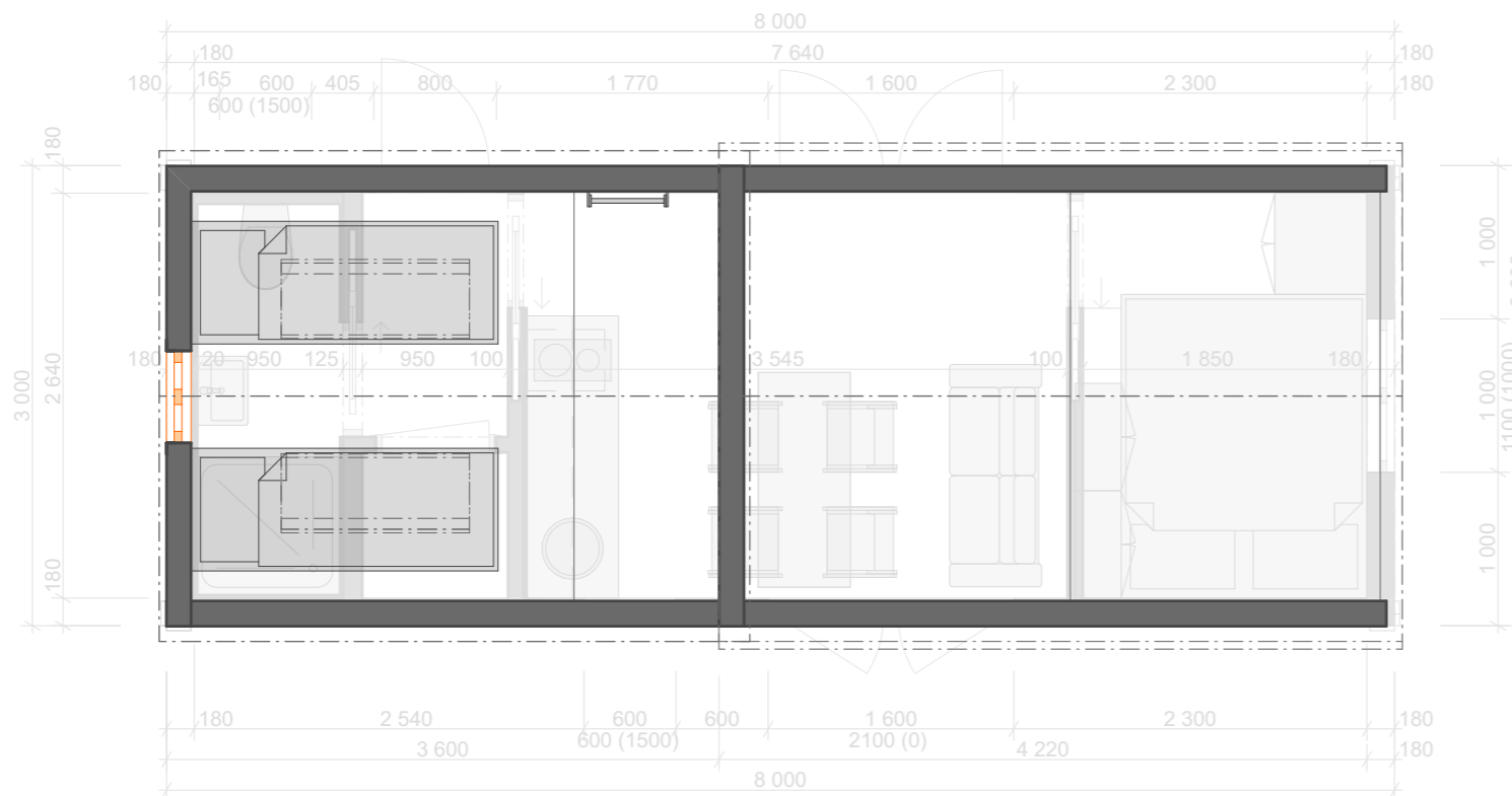
Schéma půdorysného rozvržení nástavby / patra
