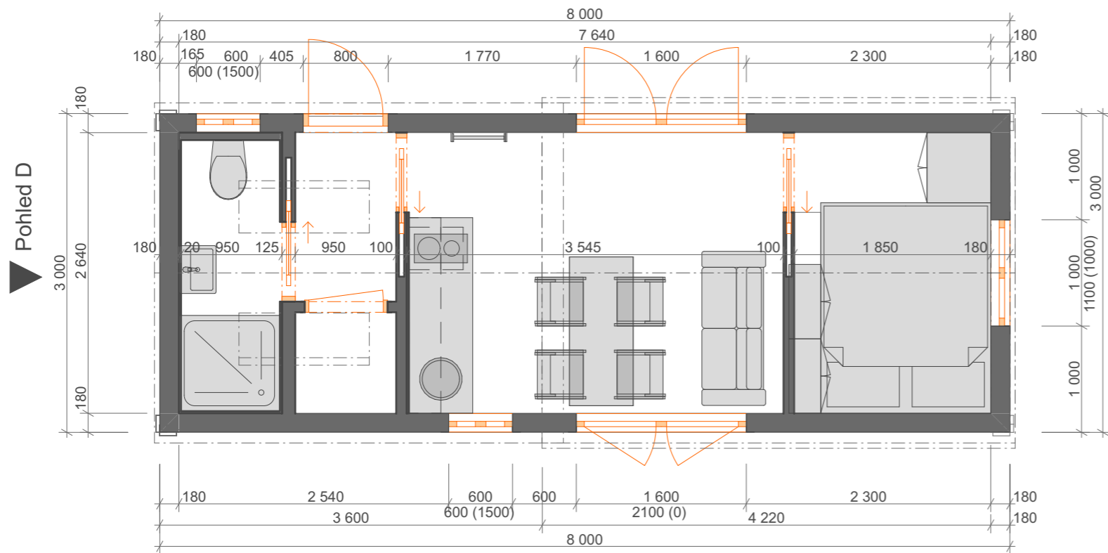
Schéma půdorysného rozvržení
