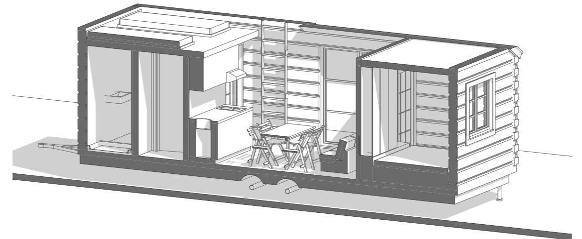
Axonometrie - řez patrem a podélný řez
