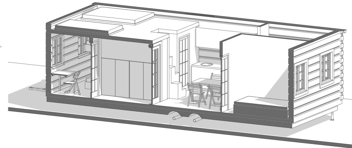
Axonometrie - řez patrem a podélný řez
