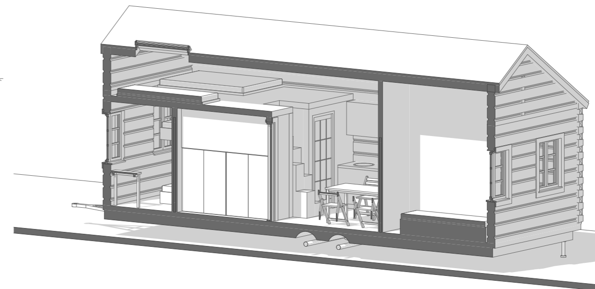
Axonometrie - podélný řez
