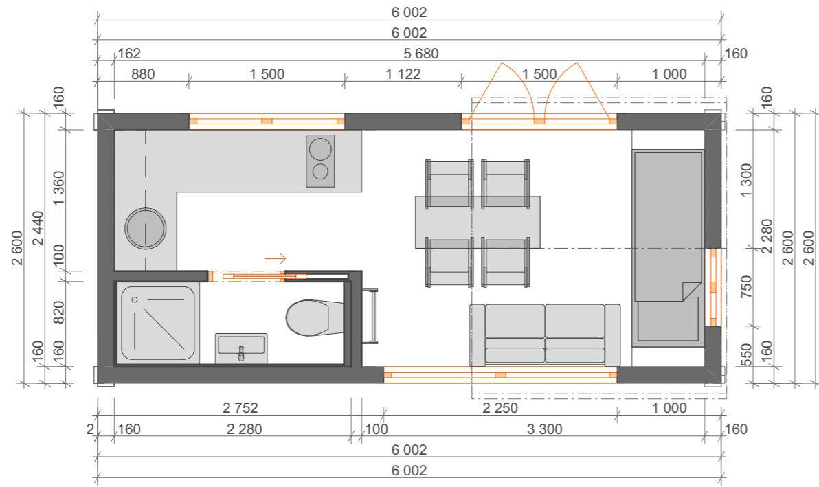
Schéma půdorysného rozvržení
