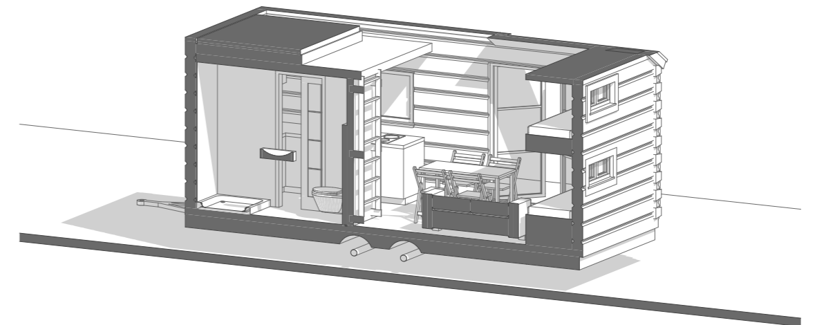
Axonometrie - řez patrem a podélný řez
