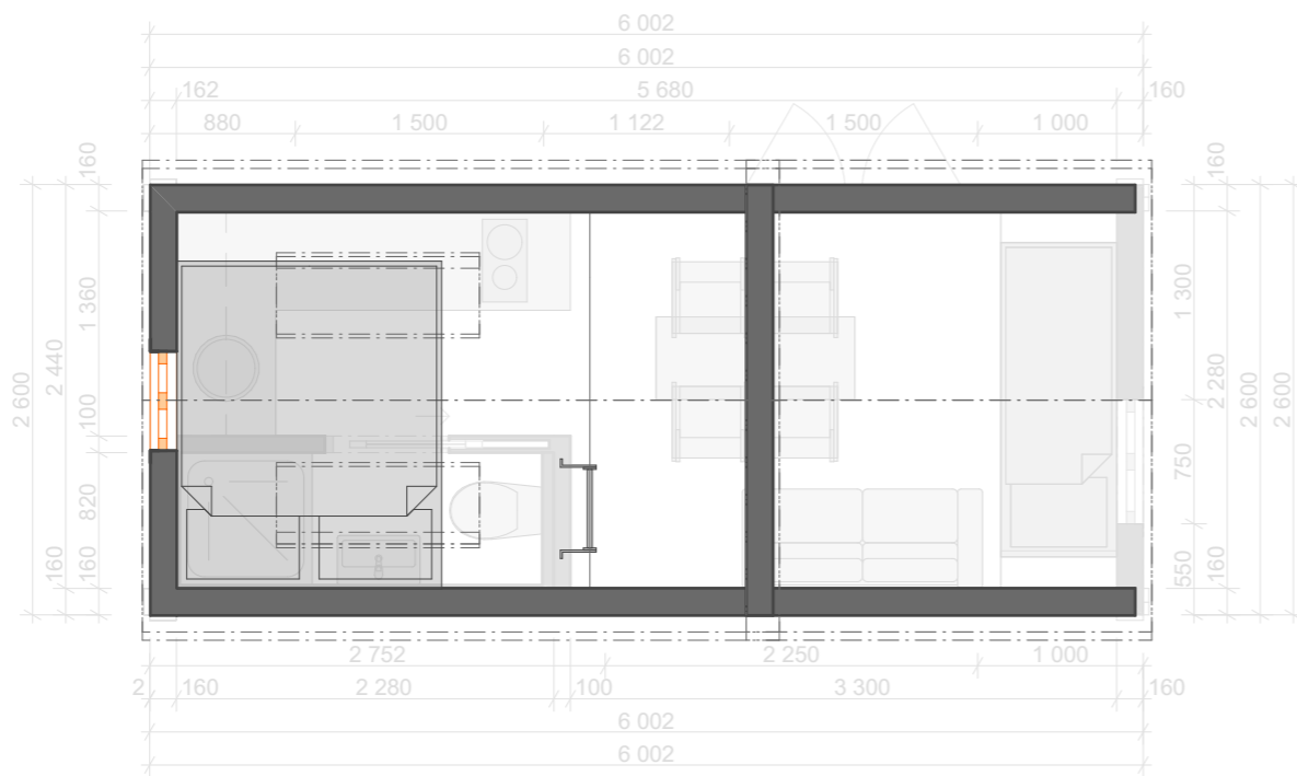
Schéma půdorysného rozvržení nástavby / patra
